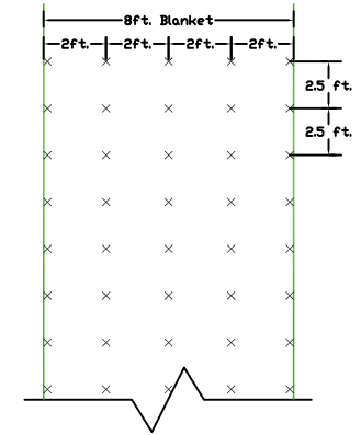
X - Indica Localización de Grapas Figura D - Vista del Plano
